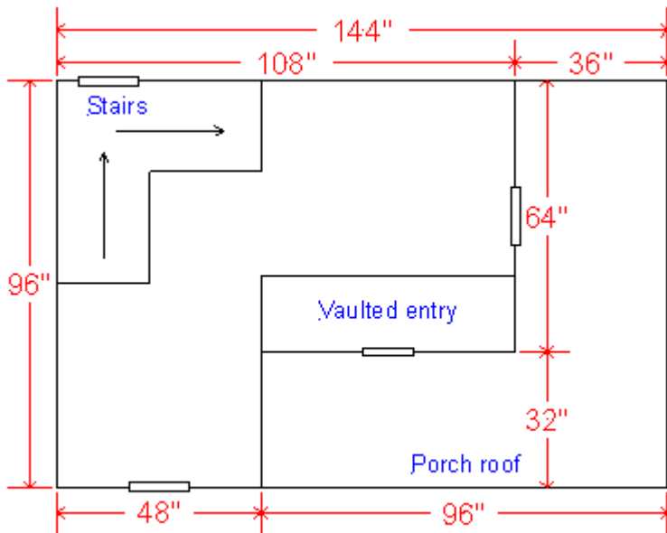
Mini Country Cottage upper floor plan
