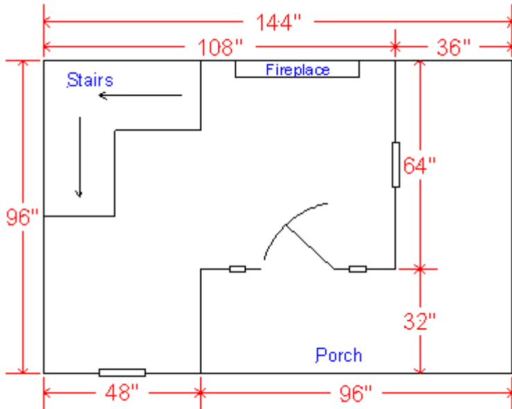
Mini Country Cottage lower floor plan
